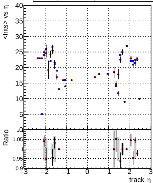
mean hits — DQM_CKF_softQCD — DQM_mkFit_SoftQCD-updated — DQM_mkFit_SoftQCD-DNNalliters
