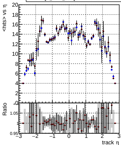
mean hit — DQM_CKF_softQCD — DQM_mkFit_SoftQCD-updated — DQM_mkFit_SoftQCD-DNNalliters
