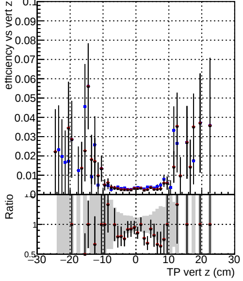
Efficiency vs TP vert z (cm) —●— DQM_CKF_softQCD —●— DQM_mkFit_SoftQCD-updated —●— DQM_mkFit_SoftQCD-DNNalliters
