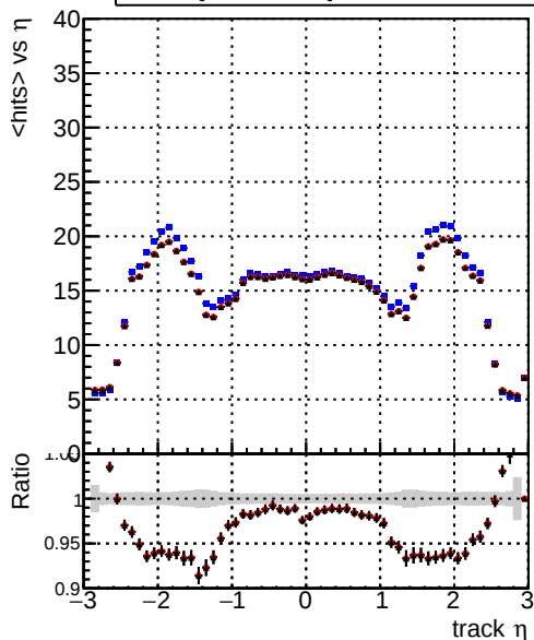
mean hits — DQM_CKF_softQCD — DQM_mkFit_SoftQCD-updated — DQM_mkFit_SoftQCD-DNNalliters
