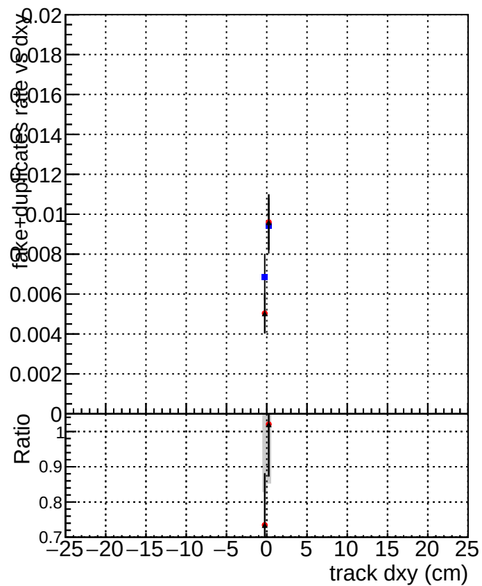
Legend: DQM_CKF_softQCD DQM_mkFit_SoftQCD-updated DQM_mkFit_SoftQCD-DNNalliters
