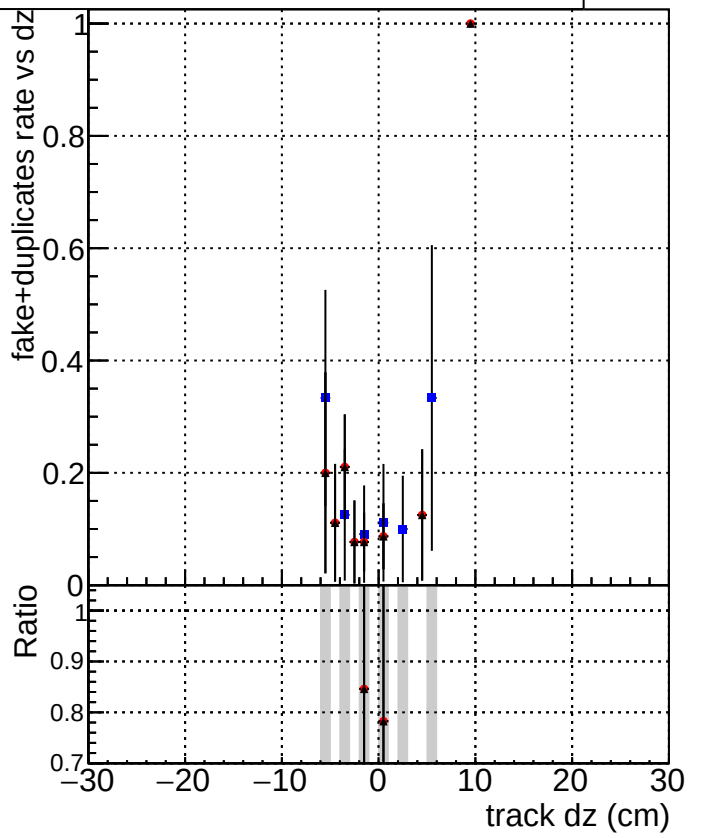
DQM_CKF_softQCD DQM_mkFit_SoftQCD-updated DQM_mkFit_SoftQCD-DNNalliters
