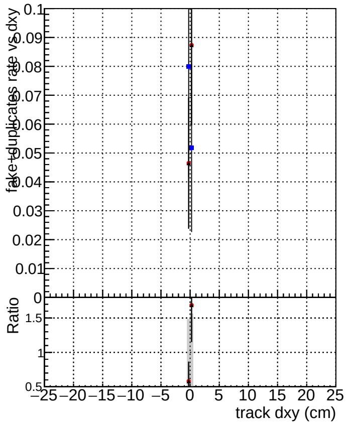
DQM_CKF_softQCD DQM_mkFit_SoftQCD-updated DQM_mkFit_SoftQCD-DNNalliters
