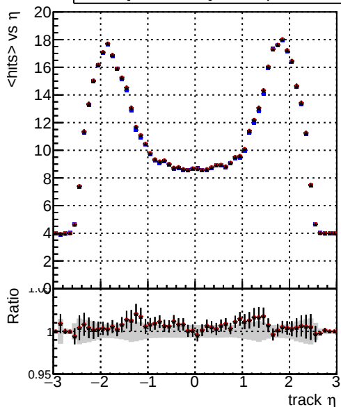
mean hits vs \eta DQM_CKF_softQCD DQM_mkFit_SoftQCD-updated DQM_mkFit_SoftQCD-DNNSqcd100
