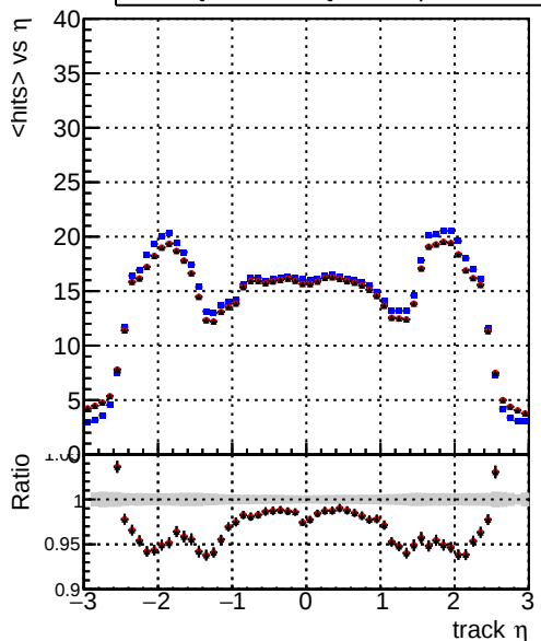
mean hits — DQM_CKF_softQCD — DQM_mkFit_SoftQCD-updated — DQM_mkFit_SoftQCD-DNNsqcd100
