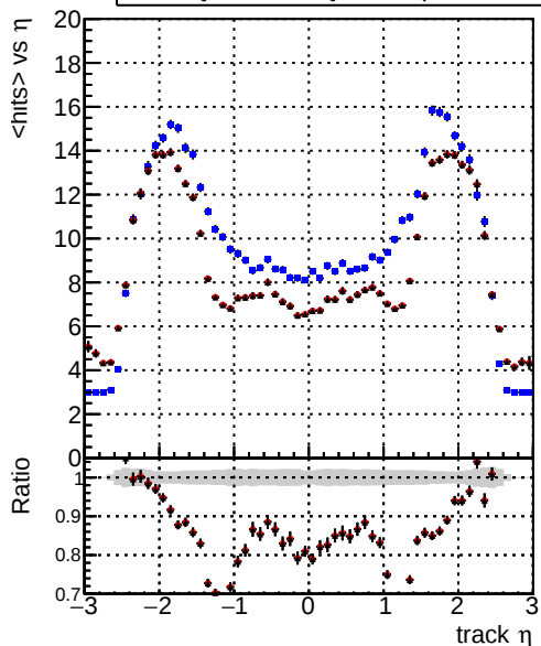
mean hits — DQM_CKF_softQCD — DQM_mkFit_SoftQCD-updated — DQM_mkFit_SoftQCD-DNNsqcd100
