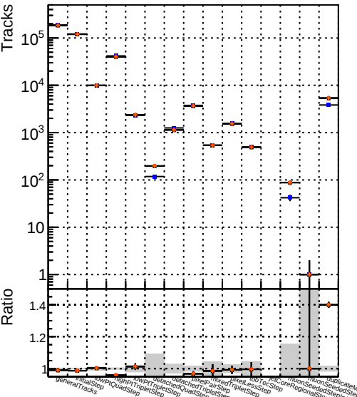
Number DQM_CKF_softQCD DQM_mkFit_SoftQCD-updated DQM_mkFit_SoftQCD-DNNsqcd100 DQM_mkFit_SoftQCD-DNNallflav
