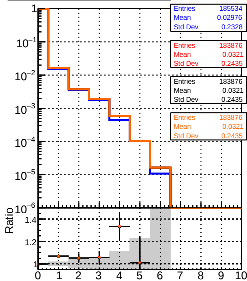
mean hit DQM_CKF_SoftQCD DQM_mkFit_SoftQCD-updated DQM_mkFit_SoftQCD-DNNsqcd100 DQM_mkFit_SoftQCD-DNNalliters
