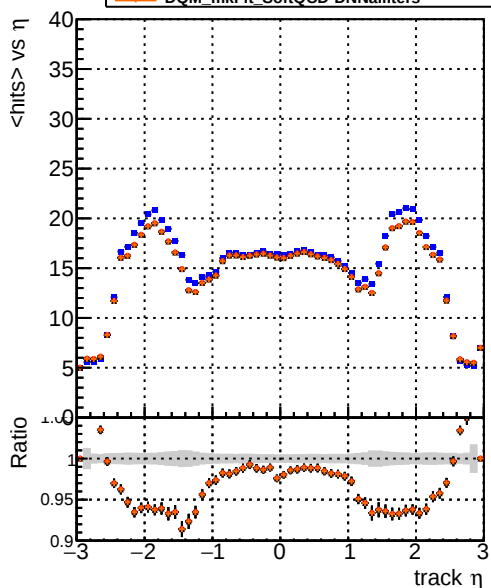
mean hits DQM_CKF_SoftQCD DQM_mkFit_SoftQCD-updated DQM_mkFit_SoftQCD-DNNsqcd100 DQM_mkFit_SoftQCD-DNNalliters
