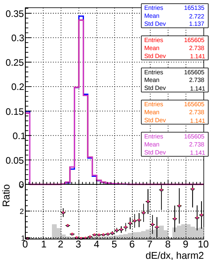
dE/dx estimator 1
