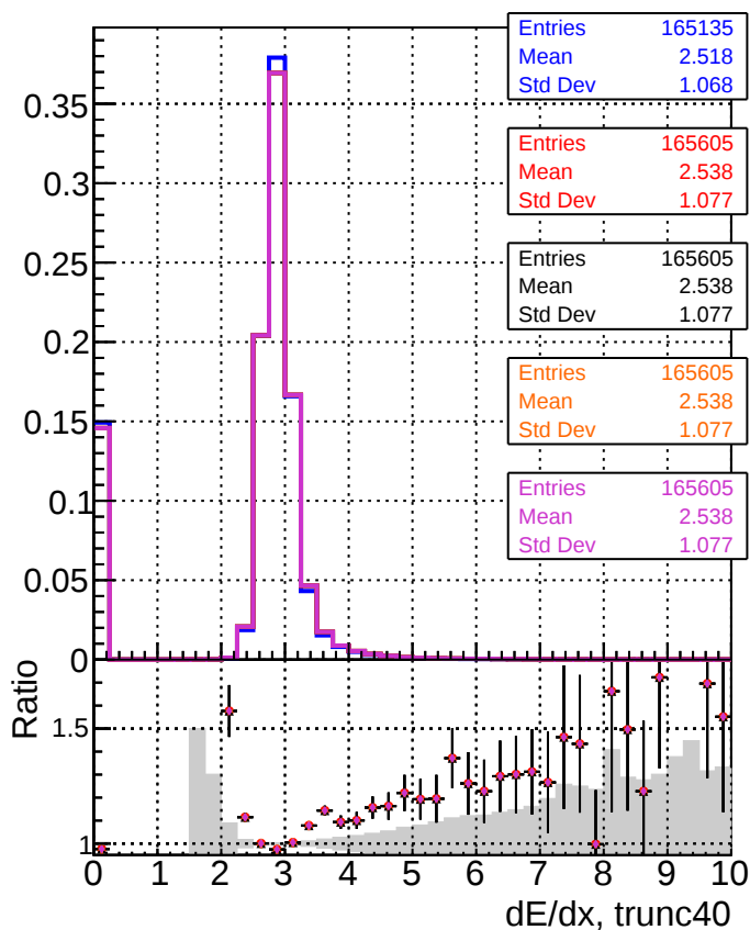
dE/dx estimator 2
