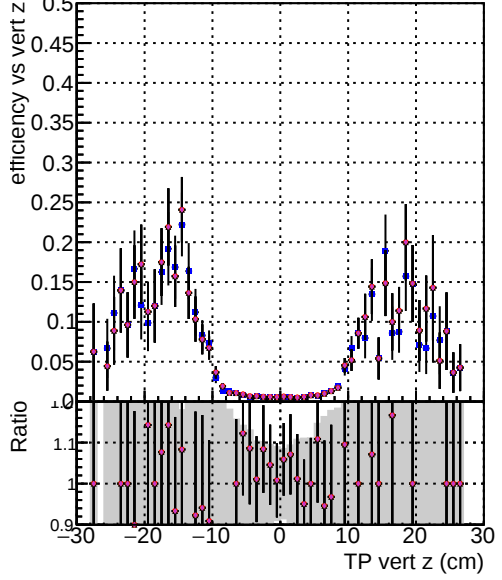
Efficiency vs vert z — DQM CKE SortOCB — DQM mkFit SortOCB — DQM mkFit SortOCB-updated — DQM mkFit SortOCB-updated-newPLDNN — DQM mkFit SortOCB-updated-TTbarDNN — DQM mkFit SortOCB-updated-DNNsgcd13
