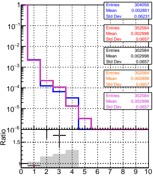
mean hit DQM_CKF_SortQCD DQM_mkFit_SortQCD-updated DQM_mkFit_SortQCD-updated-newPLDNN DQM_mkFit_SortQCD-updated-TTbarDNN DQM_mkFit_SortQCD-updated-TTbarDNN25
