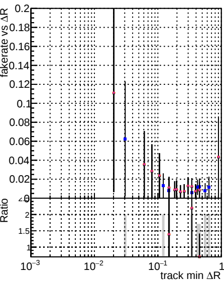
Fake rate vs ΔR(track, jet) for various models: DQM, GKE, softQCD, DQM+GKE, DQM+softQCD, DQM+GKE+softQCD, DQM+GKE+softQCD+TTbar, DQM+GKE+softQCD+TTbar+DNN25, DQM+GKE+softQCD+TTbar+DNN25+newPI, DQM+GKE+softQCD+TTbar+DNN25+newPI+DNN.
