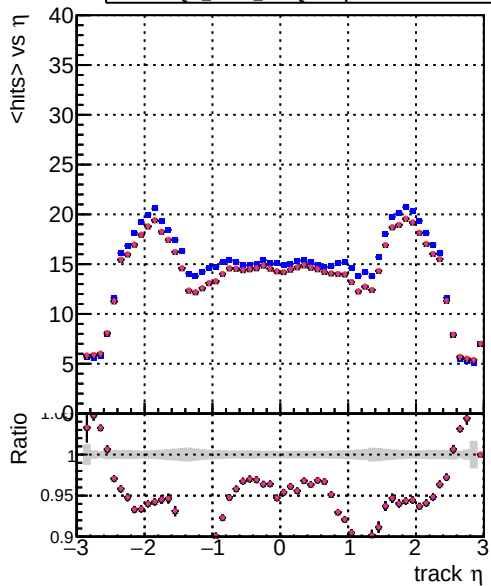
mean hit DQM_CKE_SortOCB DQM_mkFit_SortOCB-updated DQM_mkFit_SortOCB-updated-newPLDNN DQM_mkFit_SortOCB-updated-TTbarDNN DQM_mkFit_SortOCB-updated-TTbarDNN25
