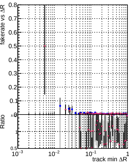
Fake rate vs ΔR(track, jet) for various models: DQM, CKF, softQCD, DQM+CKF, DQM+softQCD, DQM+CKF+softQCD, DQM+CKF+softQCD+TTbar, DQM+CKF+softQCD+TTbar+DNN25, DQM+CKF+softQCD+TTbar+DNN25+newPU, DQM+CKF+softQCD+TTbar+DNN25+newPU+DNN25.
