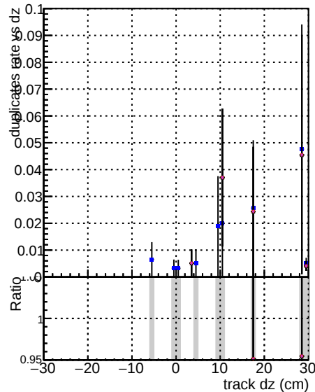
owPLDNN tbaFDNN25
