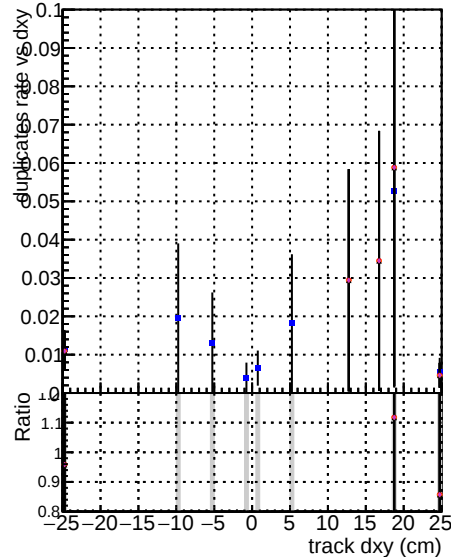
owPLDNN tbaFDNN25
