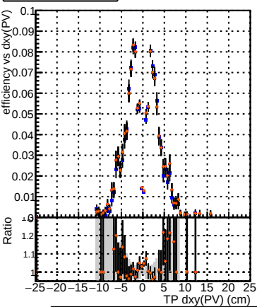
Efficiency vs Dxy(PV) Legend: DQM_CKF_softQCD DQM_mkFit_SoftQCD-updated DQM_mkFit_SoftQCD-updated-newPLDNN DQM_mkFit_SoftQCD-updated-TTbarDNN
