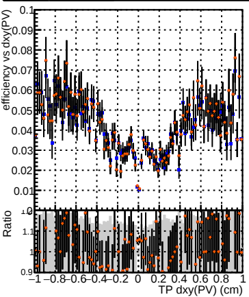
Efficiency vs Dxy(PV) Legend: DQM_CKF_softQCD DQM_mkFit_SoftQCD-updated DQM_mkFit_SoftQCD-updated-newPLDNN DQM_mkFit_SoftQCD-updated-TTbarDNN
