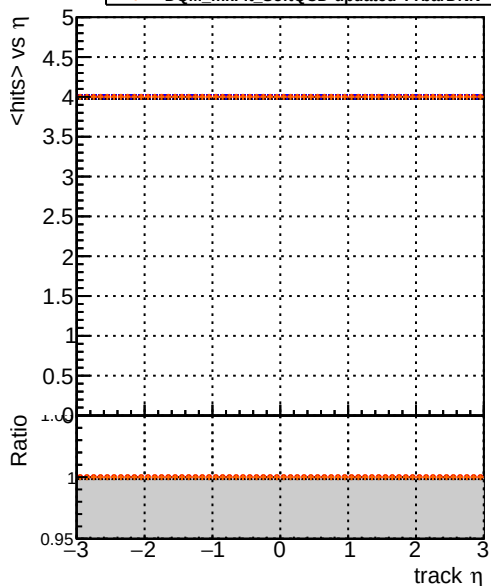
mean hits DQM_CKF_SoftQCD DQM_mkFit_SoftQCD-updated DQM_mkFit_SoftQCD-updated-newPLDNN DQM_mkFit_SoftQCD-updated-TTbarDNN
