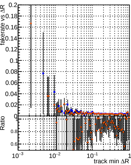
Fake rate vs \Delta R(\text{track, jet}) DQM CKE softQCD DQM mktFit softQCD-updated DQM mktFit softQCD-updated-newPI DNN DQM mktFit softQCD-updated-TTbarDNN
