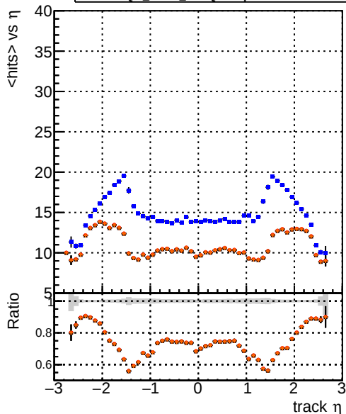
mean hit DQM_CKF_SoftQCD DQM_mkFit_SoftQCD-updated DQM_mkFit_SoftQCD-updated-newPLDNN DQM_mkFit_SoftQCD-updated-TTbarDNN
