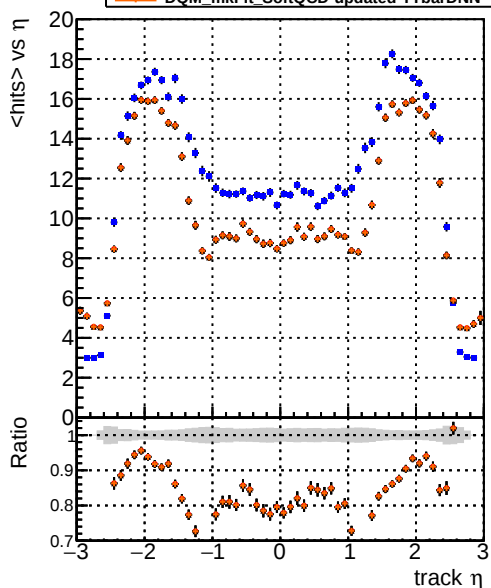
mean hit DQM_CKF_fit_SoftQCD DQM_mkFit_SoftQCD-updated DQM_mkFit_SoftQCD-updated-TPPLDNN DQM_mkFit_SoftQCD-updated-TTbarDNN
