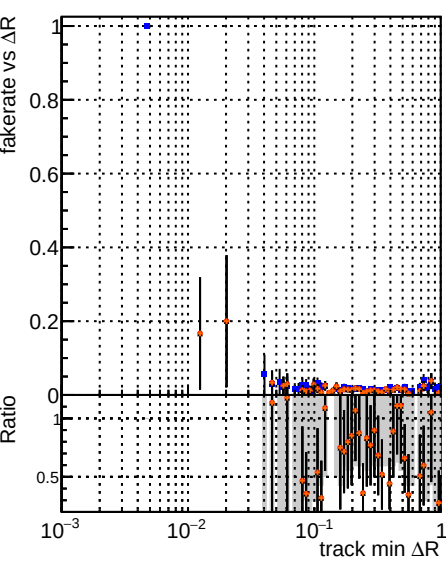
Fake rate vs \Delta R(\text{track, jet}) DQM CKE softQCD DQM mktFit softQCD-updated newPLDNN DQM mktFit softQCD-updated-TTbarDNN
