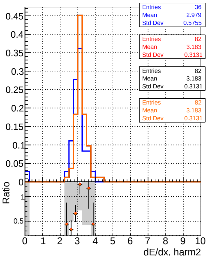
— DQM_CKF_softQCD — DQM_mkFit_SoftQCD-updated — DQM_mkFit_SoftQCD-updated-newPLDNN — DQM_mkFit_SoftQCD-updated-TTbarDNN
