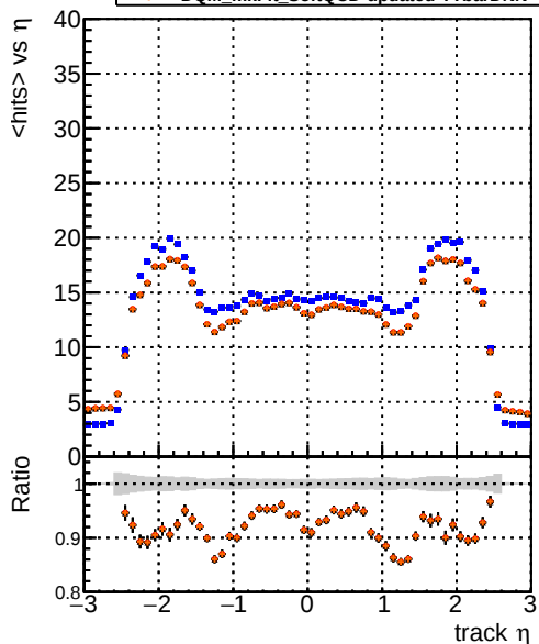
mean hit DQM_CKFit_SoftQCD DQM_mkFit_SoftQCD-updated DQM_mkFit_SoftQCD-updated-newPLDNN DQM_mkFit_SoftQCD-updated-TTbarDNN
