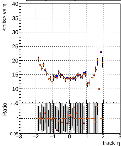
mean hit DQM_CKF_SoftQCD DQM_mkFit_SoftQCD-updated DQM_mkFit_SoftQCD-updated-newPLDNN DQM_mkFit_SoftQCD-updated-TTbarDNN
