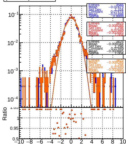
DNN pull of \theta parameter
