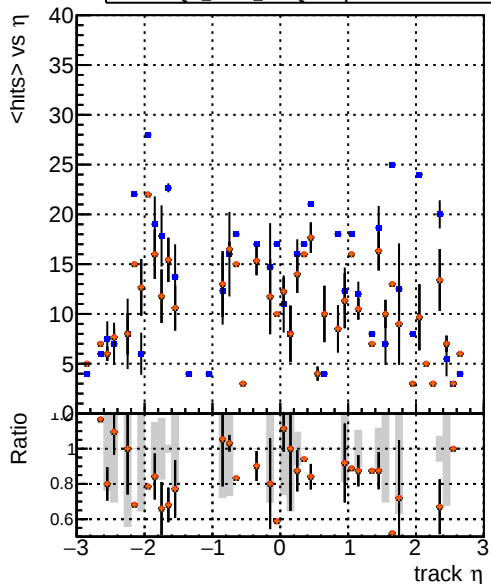
Legend: — DQM_CKF_SoftQCD — DQM_mkFit_SoftQCD-updated — DQM_mkFit_SoftQCD-updated-newPLDNN — DQM_mkFit_SoftQCD-updated-TTbarDNN mean hits
