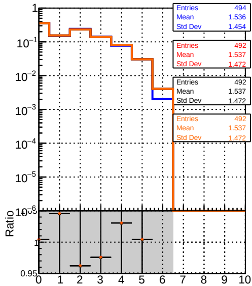
mean hit DQM_CKF_SoftQCD DQM_mkFit_SoftQCD-updated DQM_mkFit_SoftQCD-updated-newPLDNN DQM_mkFit_SoftQCD-updated-TTbarDNN
