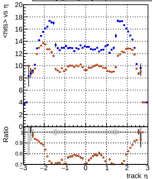
mean hit DQM_CKF_SoftQCD DQM_mkFit_SoftQCD-updated DQM_mkFit_SoftQCD-updated-newPLDNN DQM_mkFit_SoftQCD-updated-TTbarDNN
