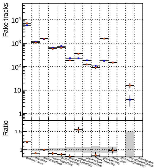
Number Model 1 DQM_mklFit_SoftQCD-updated-newPLDNN 2 DQM_mklFit_SoftQCD-updated-TTbarDNN
