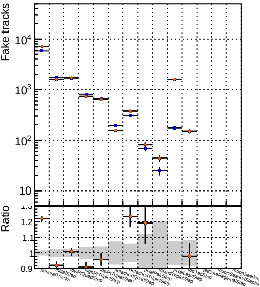
Number Model Updated 1 DQM_mkFit_SoftQCD-updated-newPLDNN 2 DQM_mkFit_SoftQCD-updated-TTbarDNN
