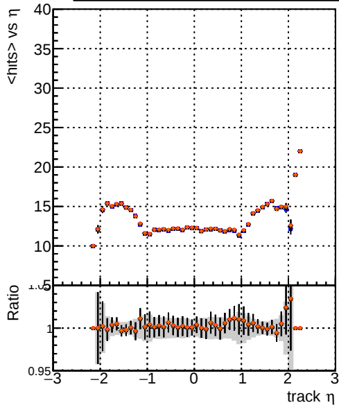
DQM_CKF_SoftQCD DQM_mkFit_SoftQCD-updated DQM_mkFit_SoftQCD-updated-newPLDNN DQM_mkFit_SoftQCD-updated-TTbarDNN mean hit
