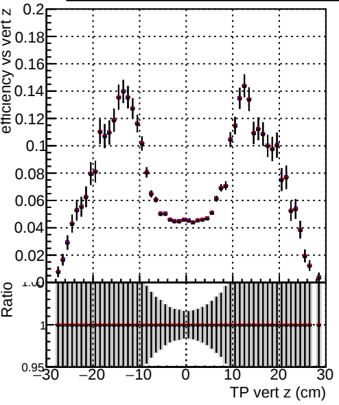
Efficiency vs TP vert z (cm) Legend: DQM_mkFit_SoftQCD-updated DQM_mkFit_SoftQCD-updated-newPLDNN DQM_mkFit_SoftQCD-updated-TTbarDNN
