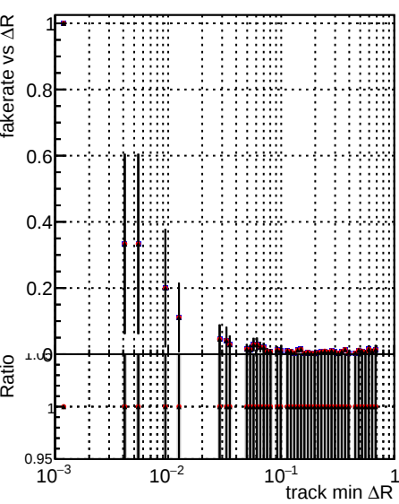
Legend: — DQM MkFit SoftQCD-updated — DQM MkFit SoftQCD-updated-newPLDNN — DQM MkFit SoftQCD-updated-TTbarDNN
