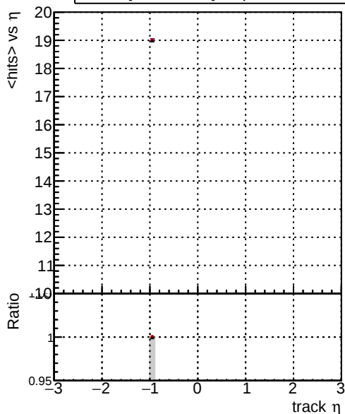
mean hit — DQM_mkFit_SoftQCD-updated — DQM_mkFit_SoftQCD-updated-newPLDNN — DQM_mkFit_SoftQCD-updated-TTbarDNN
