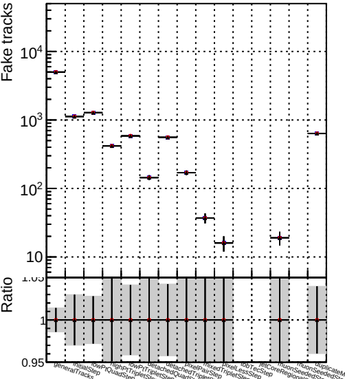
Number —■— DQM_mkFit_SoftQCD-updated —●— DQM_mkFit_SoftQCD-updated-newPLDNN —▲— DQM_mkFit_SoftQCD-updated-TTbarDNN
