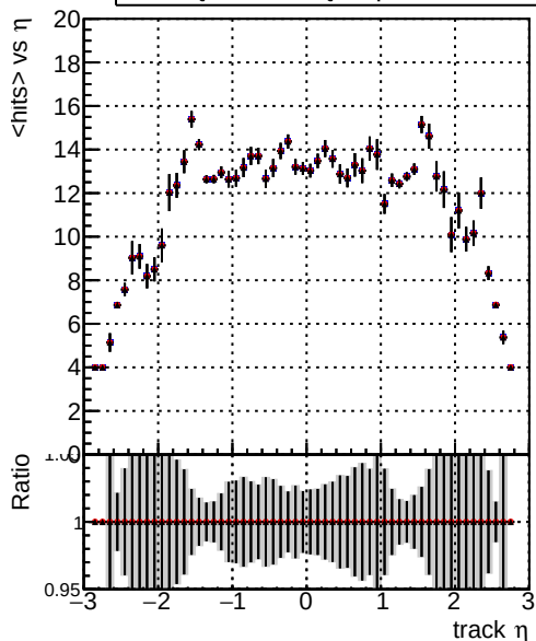
mean hits vs \eta DQM_mkFit_SoftQCD-updated DQM_mkFit_SoftQCD-updated-newPLDNN DQM_mkFit_SoftQCD-updated-TTbarDNN
