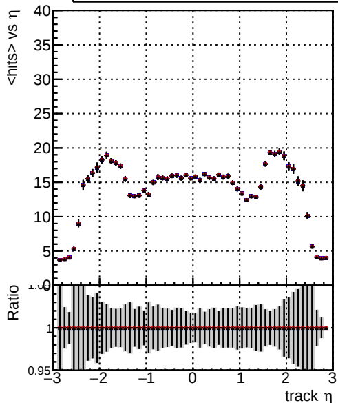
mean hits — DQM_mkFit_SoftQCD-updated — DQM_mkFit_SoftQCD-updated-newPLDNN — DQM_mkFit_SoftQCD-updated-TTbarDNN
