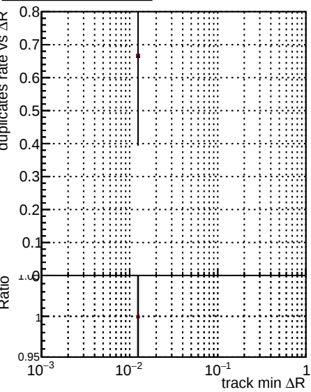
DOM_mkFit_SoftQCD-updated DOM_mkFit_SoftQCD-updated-newPLDNN DOM_mkFit_SoftQCD-updated-TTbarDNN
