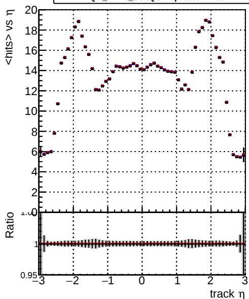
mean hits vs \eta DQM_mkFit_SoftQCD-updated DQM_mkFit_SoftQCD-updated-newPLDNN DQM_mkFit_SoftQCD-updated-TTbarDNN
