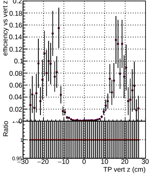
Efficiency vs. TP vert z — DQM_mkFit_SoftQCD-updated — DQM_mkFit_SoftQCD-updated-newPLDNN — DQM_mkFit_SoftQCD-updated-TTbarDNN
