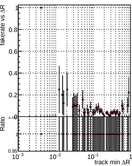
Legend: - DQM_mkFit_SoftQCD-updated - DQM_mkFit_SoftQCD-updated-newPLDNN - DQM_mkFit_SoftQCD-updated-TTbarDNN
