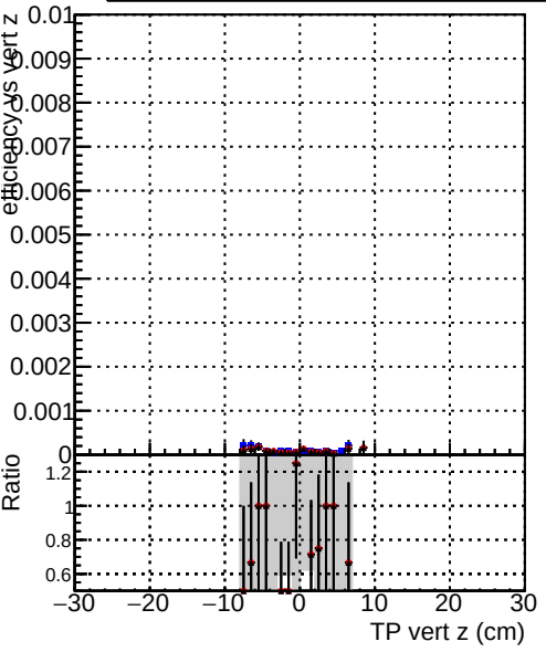
Efficiency vs vertpos DQM_CKF_softQCD DQM_mkFit_SoftQCD-updated DQM_mkFit_SoftQCD-updated-newPLDNN
