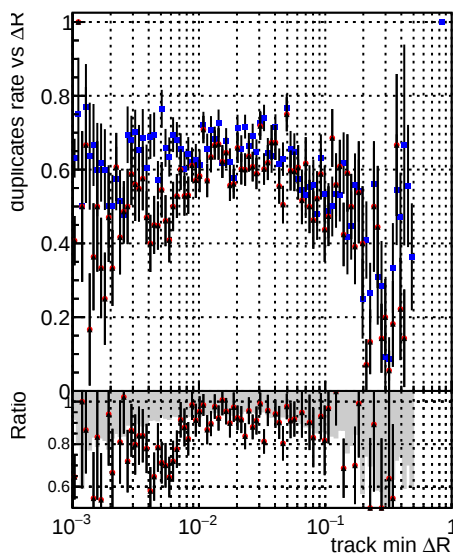
—●— DQM_CKF_softQCD —●— DQM_mkFit_SoftQCD-updated —●— DQM_mkFit_SoftQCD-updated-newPLDNN
