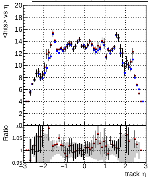
mean hits — DQM_CKF_softQCD — DQM_mkFit_SoftQCD-updated — DQM_mkFit_SoftQCD-updated-newPLDNN
