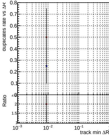
Legend: DQM_CKF_softQCD DQM_mkFit_SoftQCD-updated DQM_mkFit_SoftQCD-updated-newPLDNN
