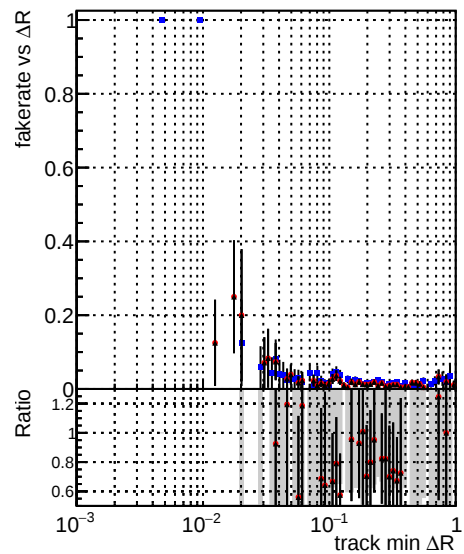
Legend: DQM_CKF_softQCD DQM_mkFit_SoftQCD-updated DQM_mkFit_SoftQCD-updated-newPLDNN
