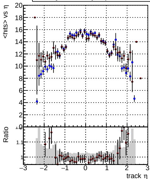
mean hits vs \eta DQM_CKF_softQCD DQM_mkFit_SoftQCD-updated DQM_mkFit_SoftQCD-updated-newPLDNN
